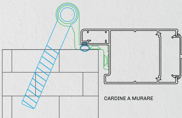
COD. TEL 50 TELAIO CON ALETTA DA mm 50
