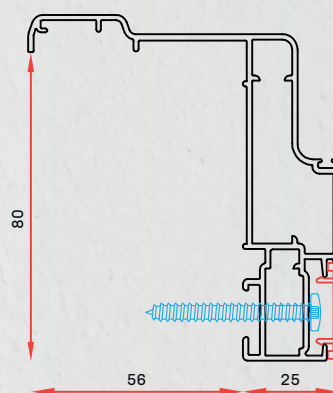
COD. GX 03 TELAIO STORICO CON CARTERINO COPRI FISSAGGIO
